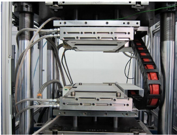
100 トンプレス機 誘導金型加熱装置
