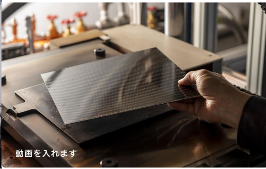
誘導 H&C 熱盤兼プレス金型/CFRP 成形品
